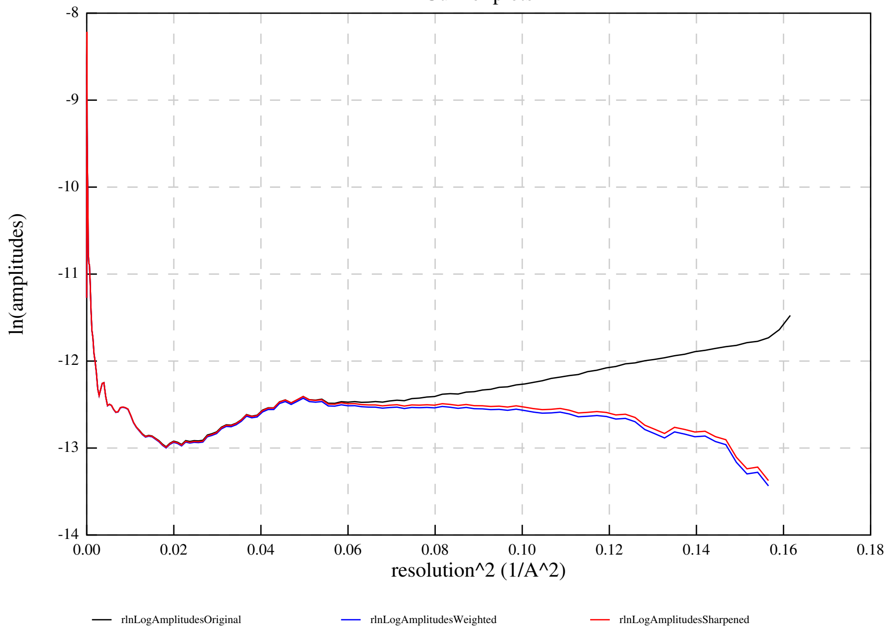
Guinier plots
